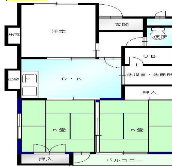
間取り図
