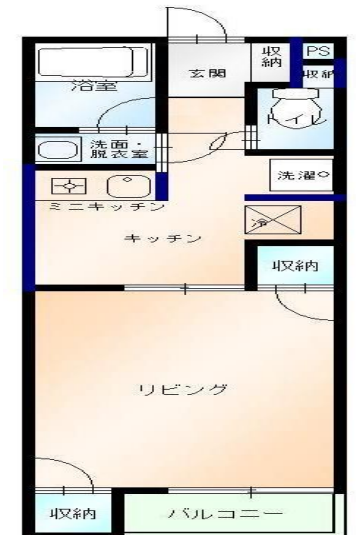
間取り図
